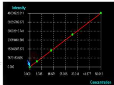
ICP-AES
